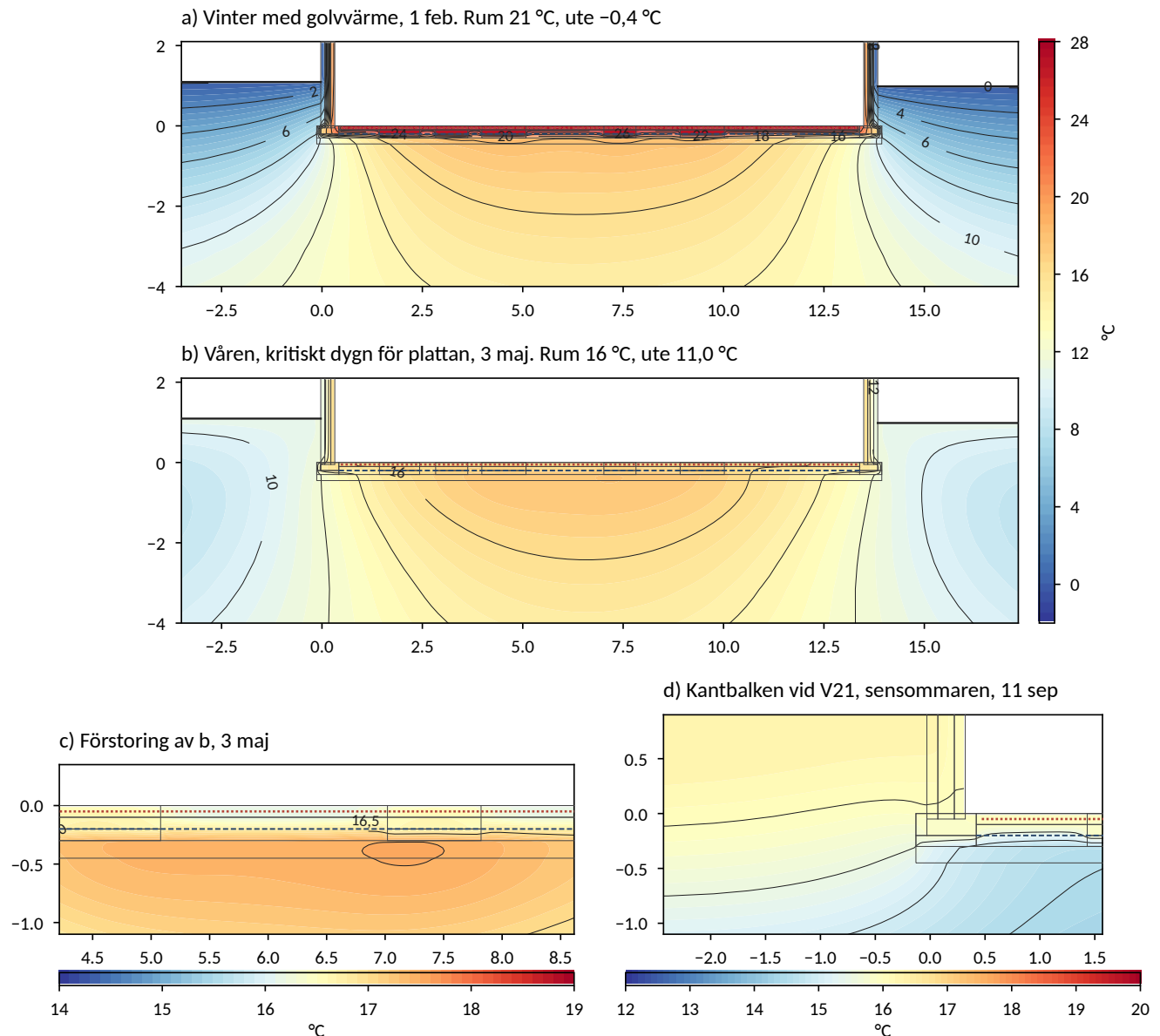
Figur 3: Temperaturfält i grundfallet. Isothermer med 2 K avstånd i a och b, 0,5 K i c och d. I c är marken under plattan och plintarna varmare än betongen.
