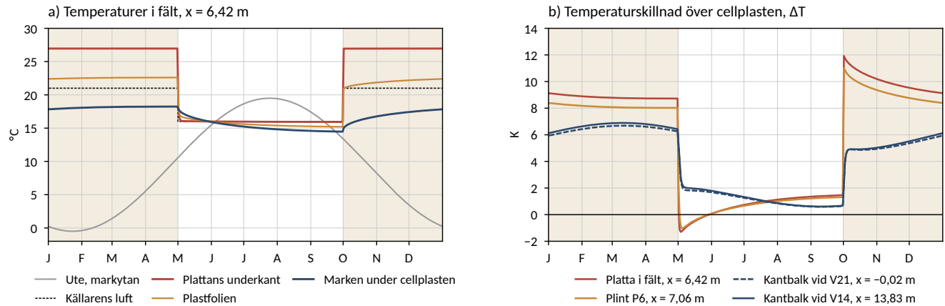
Figur 2: Grundfallet under året. a) Temperaturlinjer i fält där \Delta T är minst. b) \Delta T där den är minst för plattan i fält, plintarna och kantbalkarna. Skuggat: golvvärme.
