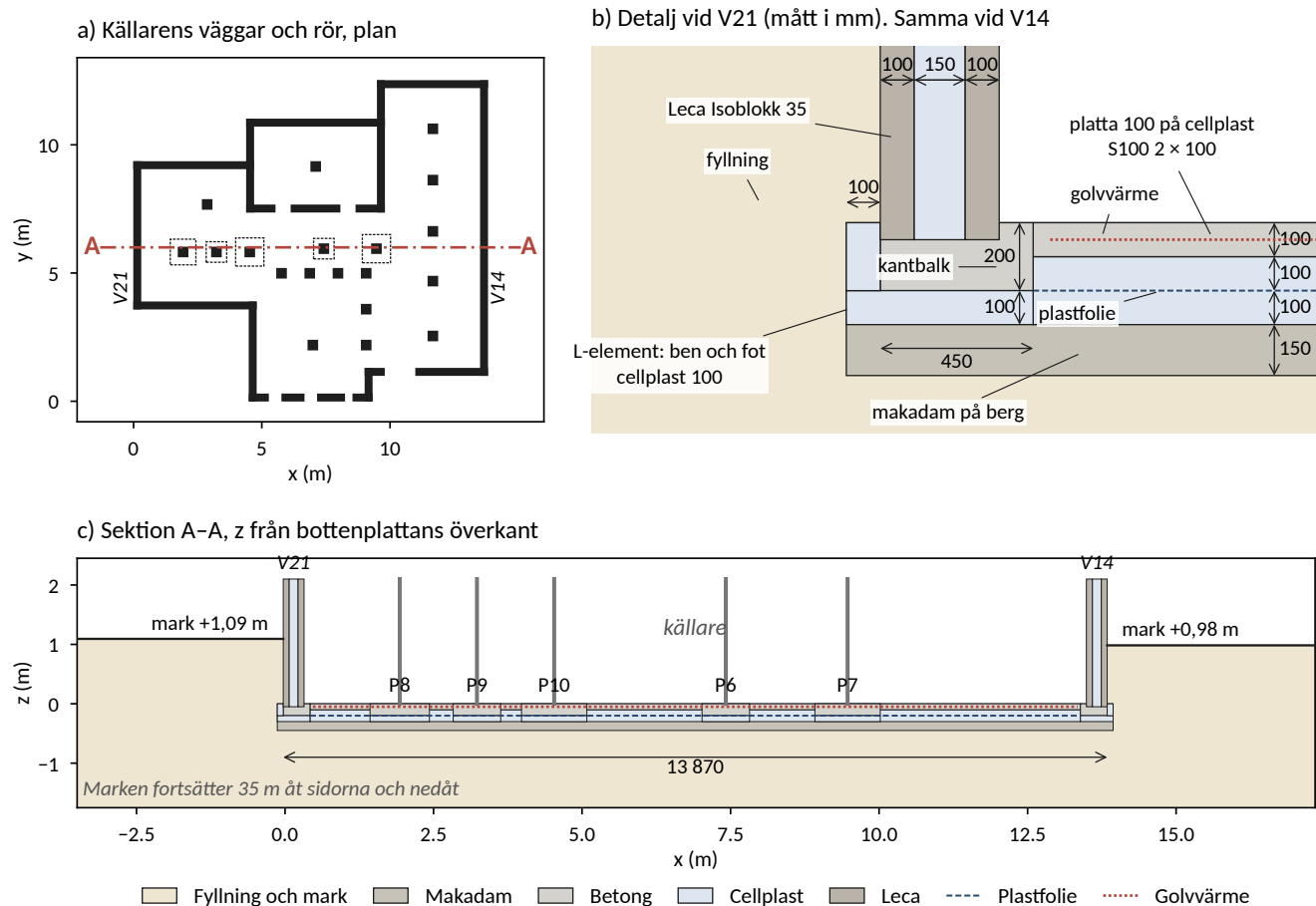
Figur 1: Sektion A-A med beräkningsmodellens geometri. Koordinater som i K-05. z räknas från bottenplattans överkant.
